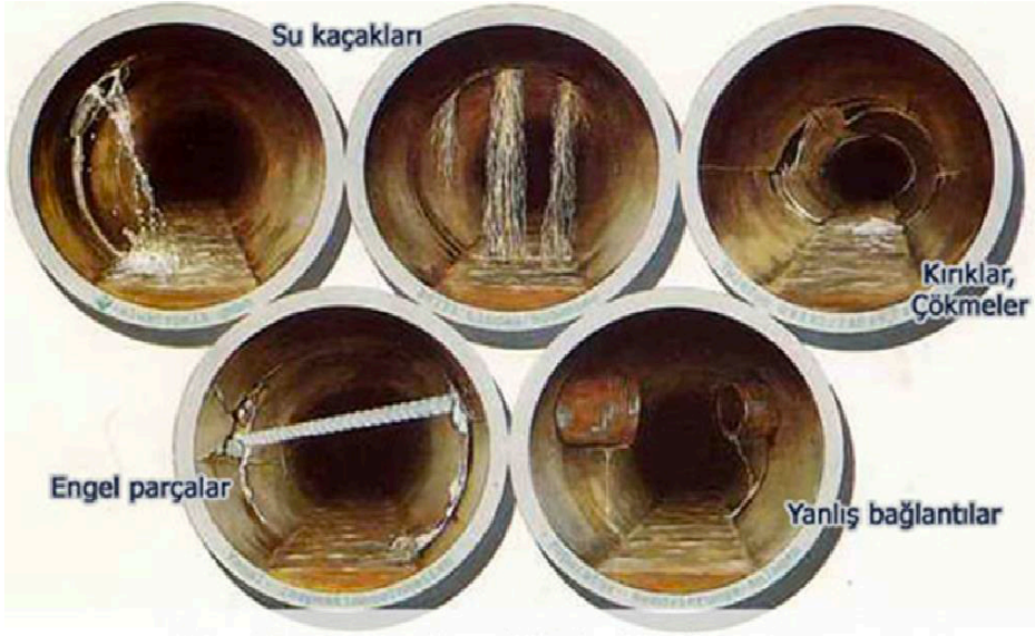
Şekil 3.3. Kanalizasyon Sisteminde Muhtemel Kusurlar
